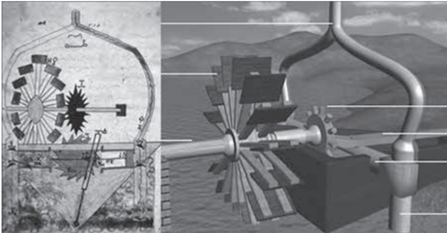
Slika 6. (lijevo) – Al-Jazarijeva dvocilindrična usisna pumpa i ilustracija radilice. – (desno) 3D animirana slika usisne pumpe.
