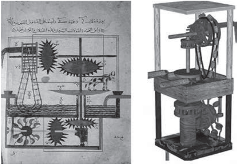
Slika 5. (lijevo) – Stranica rukopisa iz 13. vijeka prikazuje mašinu za podizanje vode, koju je dizajnirao Al-Jazari u kopiji rukopisa koja se čuva u biblioteci Topkapi Saraya u Istanbulu.
